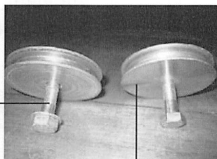
滑車軸の摩耗
